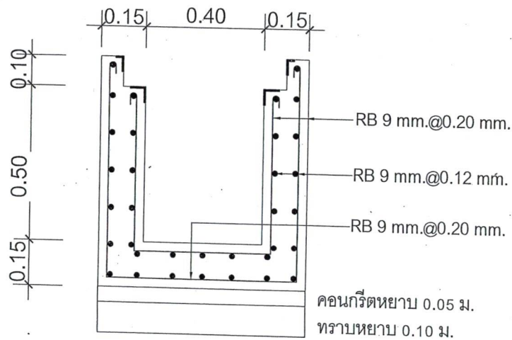
แบบขยายวางระบายนํ้า
