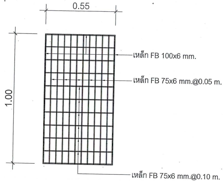
แบบขยายฝาดะแกรงเหล็ก
