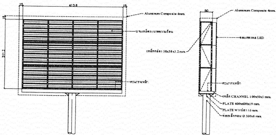
รูปขยายโครงสร้างด้านหลัง NOT TO SCALE
