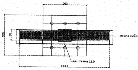
รูปลายคานบน NOT TO SCALE
